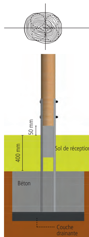
Piètements d'ancrage pour poteaux en bois douglas
