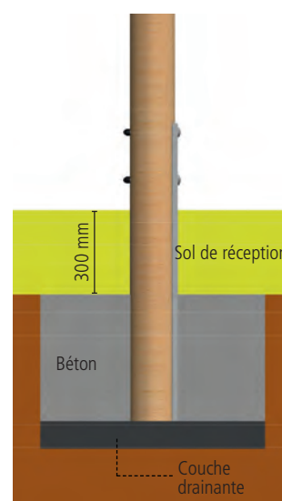
Attelles en acier pour poteaux en robinier et en chêne (1 attelle latérale pour le chêne, 2 attelles pour le robinier)
