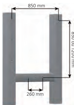
Schéma type pour un pont en V avec corde centrale Hauteur garde-corps : 850 ou 1200 mm
