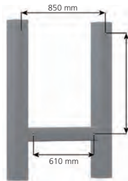
Schéma type pour un pont en U avec passerelle Largeur utile : 75 cm Hauteur garde-corps : 900 ou 1200 mm
