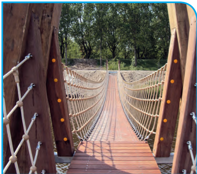
HUCK Torimex (Pays-Bas) Pont à lattes en 2 parties (25.70 m et 11.30 m) avec piliers bois intermédiaires
