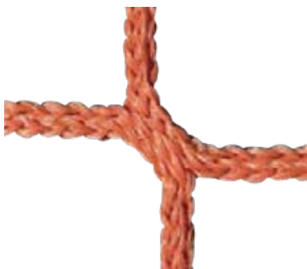
n° 212 rouge, sans nœuds Polypropylène haute résistance, ø 5 mm
