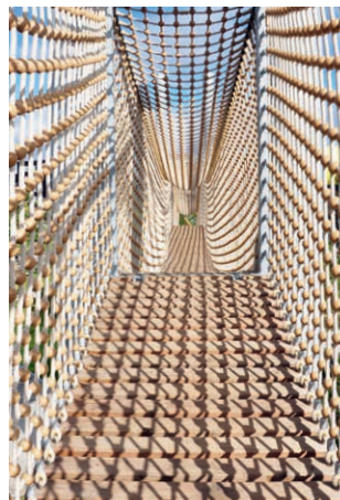
Tunnel en câble Hercule, maille 125 x 125 mm, passage en lattes de bois
