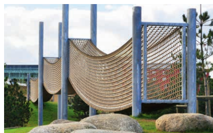
Tunnel en câble Hercule avec passage en lattes de bois, longueur 40 m
