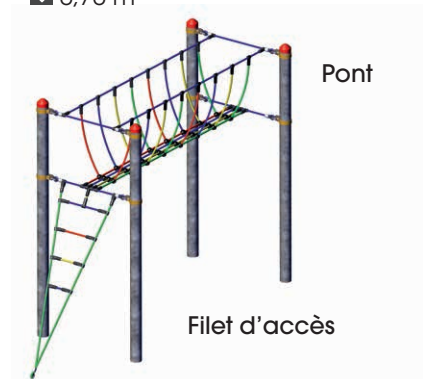
Pont et Filet d'accès Vario
