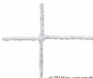
n° 201 blanc, sans nœuds, polypropylène haute résistance, \varnothing 1.8 mm
