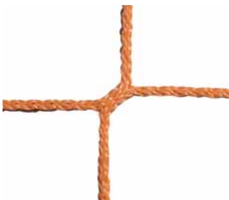
n° 205 orange, sans nœuds Polypropylène haute résistance, ø 2.8 mm
