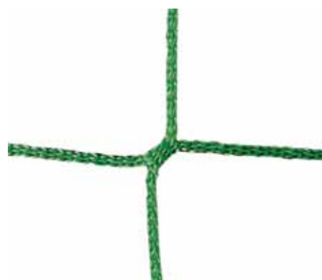
n° 200 vert foncé, sans nœuds Polypropylène haute résistance, ø 2.3 mm
