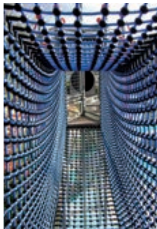
Tunnel en câble Hercule, rectangulaire, maille 125 x 125 mm
