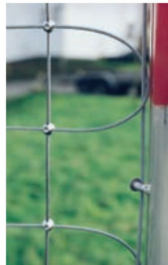
Détail du montage anti-vol par câble transféré
