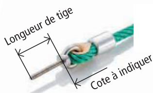
Anneau et tige filetée Inox Réf. 455B M8/M10/M12
